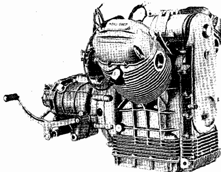
Fig. 3 - Motore completo di cambio
