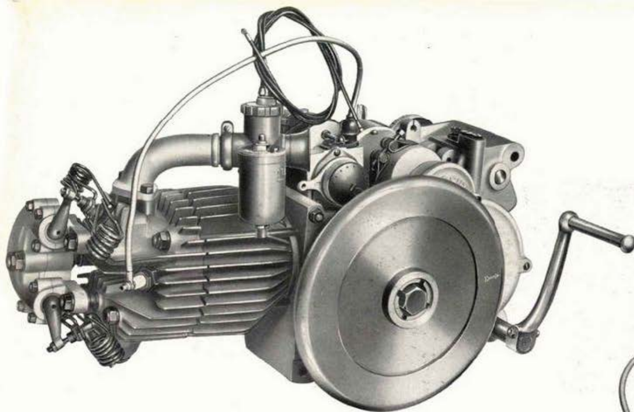
Fig. 4 - Lato volano
