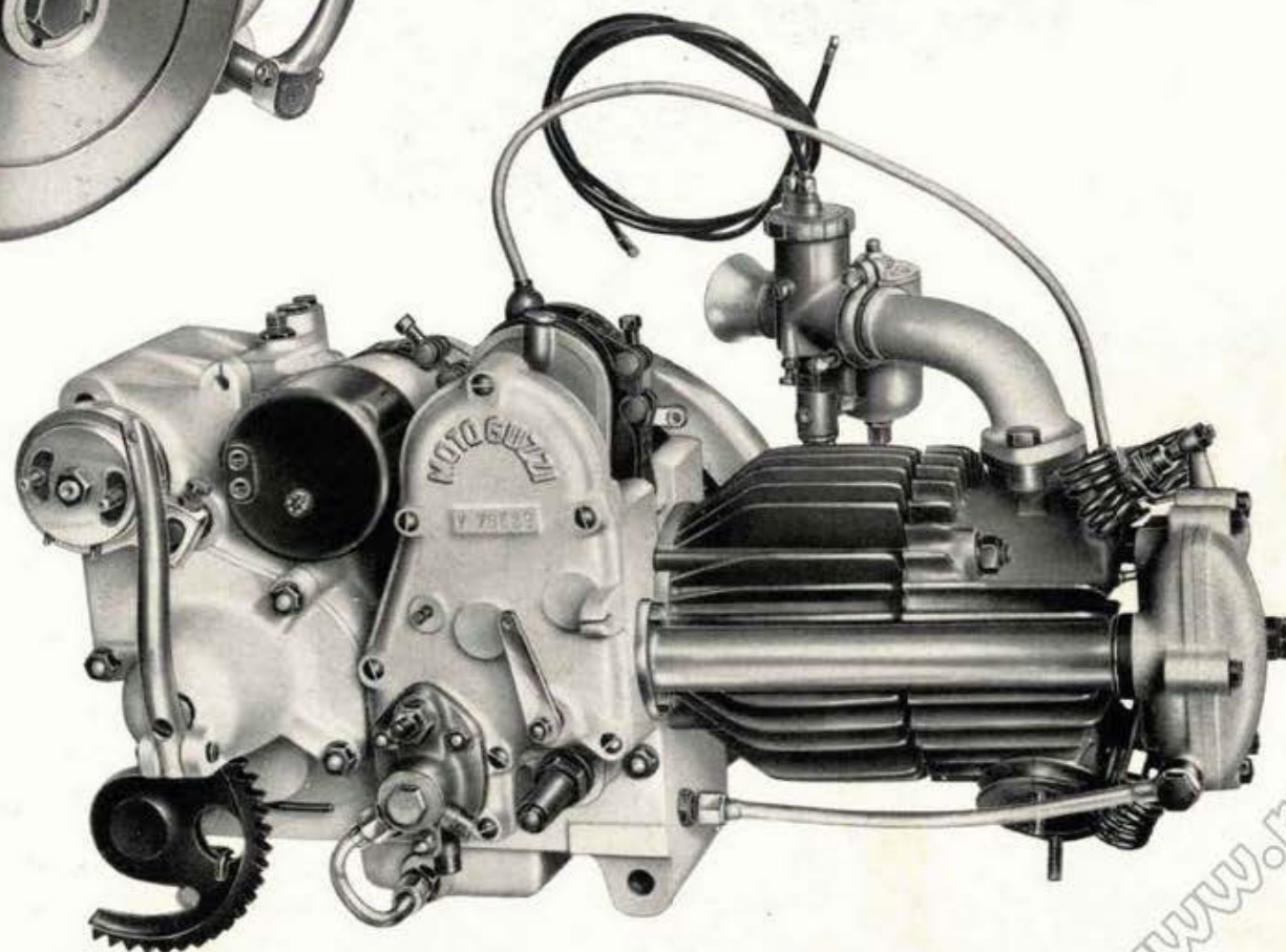
Fig. 5 - Lato distribuzione
